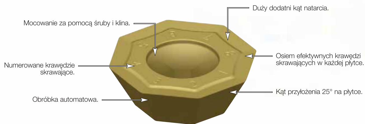
Płytki OF.T06/OF.T07
